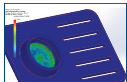
Spannungsverteilung eines Kunststoffteils, das einer externen Belastung gepaart mit Gussform-Restspannungen unterliegt
