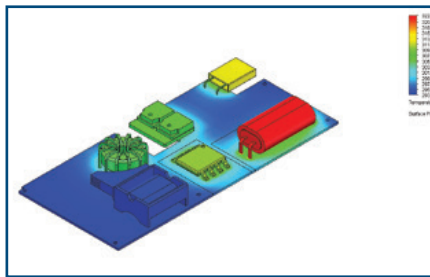
Temperaturverteilung einer CFD-Analyse in SOLIDWORKS Flow Simulation
