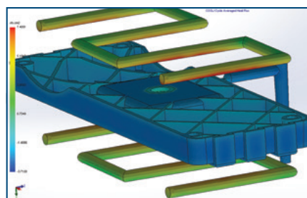
Wärmefluss einer SOLIDWORKS Plastics Kühlsimulation des Hohlraums, der Kühlkanäle und Gussform
