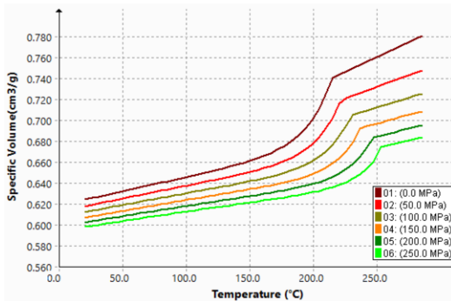
Gleiche Materialsorte aktualisiert mit generischen PVT-Daten (2022)
